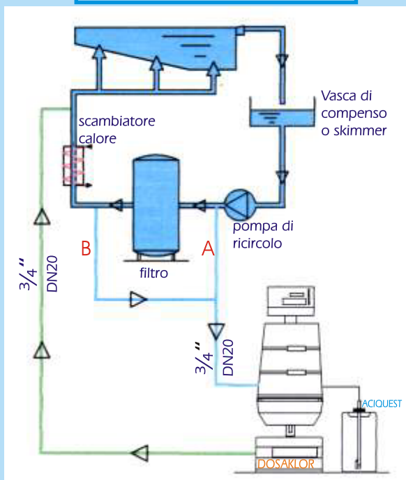
Schema d'installazione
